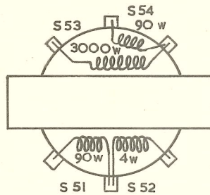
UITGANGSTRAFO GK 512 80
