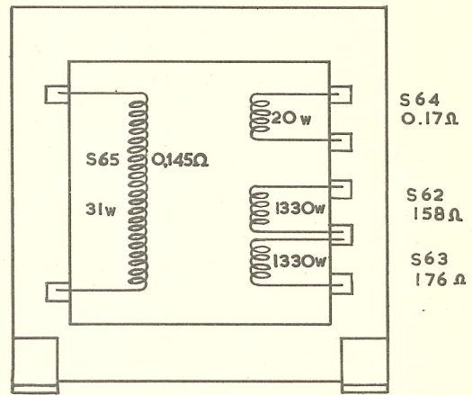
VOEDINGSTRAFO GK 512 74
